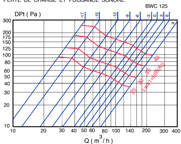
PERTE DE CHARGE ET PUISSANCE SONORE.
