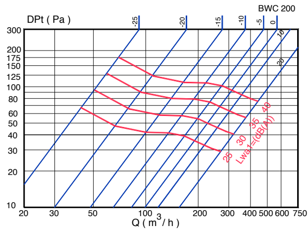
PERTE DE CHARGE ET PUISSANCE SONORE.
