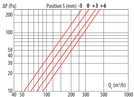
BOC - BMI Ø 160
