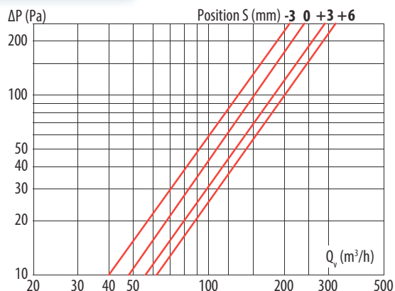
BOC - BMI Ø 125
